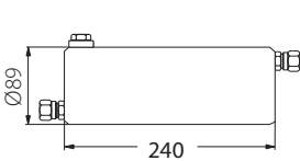
Охладитель импульса давления V1
