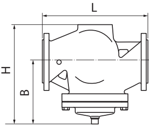
VFG-2R DN150-250
